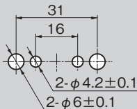
패널 구멍 치수 Panel drilling dimensions
