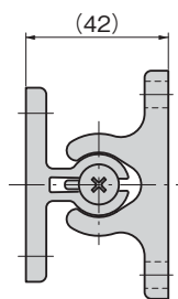
맞물림 높이 참고 Engagement height reference
