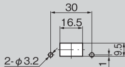
패널 구멍 치수 Panel drilling dimensions
