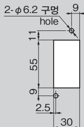
패널 구멍 치수 Panel drilling dimensions
