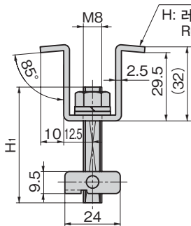
누름 플레이트 Holding plate
