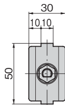
가대 구멍 치수 Support drilling dimensions
