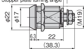
스톱퍼 회전 각도 90° Stopper plate turning angle
