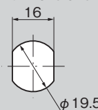
패널 구멍 치수 Panel drilling dimensions
