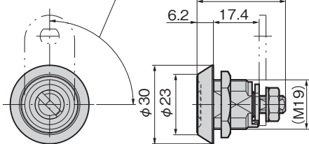
스톱퍼 회전 각도 90° Stopper plate turning angle (33.5)
