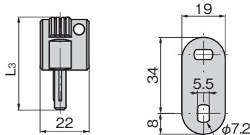
패널 구멍 치수 Panel drilling dimensions
