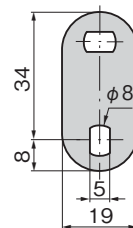
판 두께 t=3.2 Plate thickness
