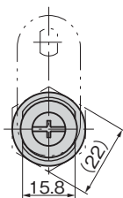
패널 구멍 치수 Panel drilling dimensions
