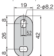
패널 구멍 치수 Panel drilling dimensions
