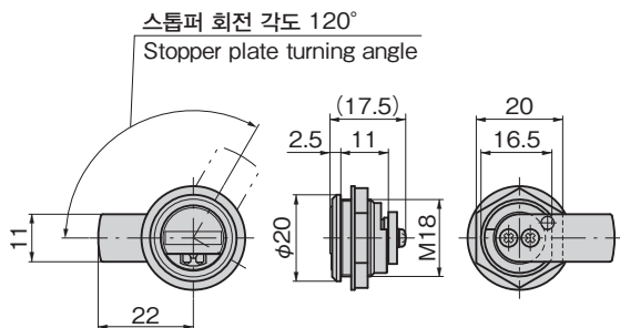
키 No.JD0494 Key
