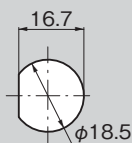
패널 구멍 치수 Panel drilling dimensions
