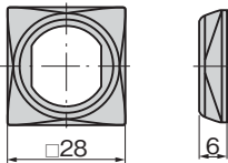
스톱퍼 회전 각도 90° Stopper plate turning angle
