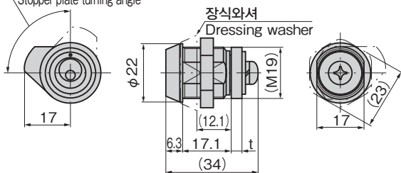
스톱퍼 회전 각도 90° Stopper plate turning angle
