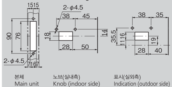
패널 구멍 치수 Panel drilling dimensions
