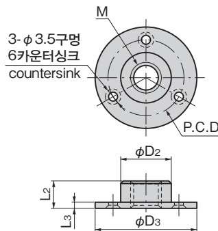
[ KC-1270-W 캐치 플레이트 ] [ Catch plate ]
