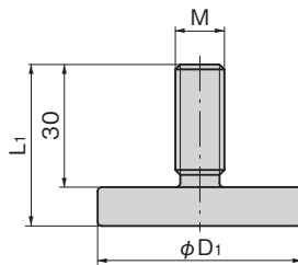
[ KC-1270 본체 ] [ Main body ]
