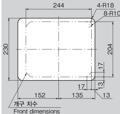
패널 구멍 치수 Panel drilling dimensions
