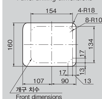
패널 구멍 치수 Panel drilling dimensions
